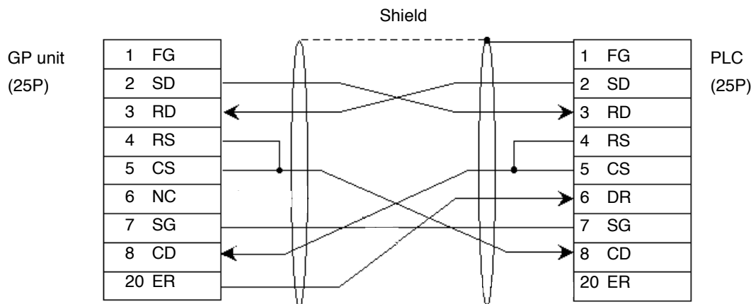
Cable Diagram 8 (RS-232C)
